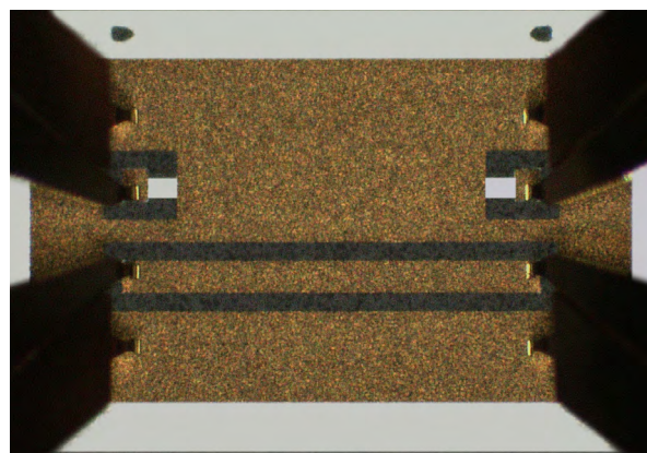
2つの向かい合ったGSSG TITAN™デュアルプローブを10μmの垂直オーバートラベルでThru (Adj Load)標準器に触れた後、プローブを離れた時の写真。
