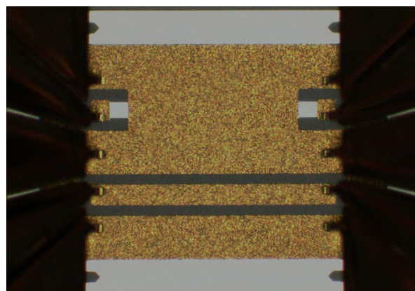
2つの向かい合ったGSGSG TITAN™デュアルプローブを10μmの垂直オーバトラベルでThru(Adj Load)標準器に触れた後、プローブを離れた時の写真
