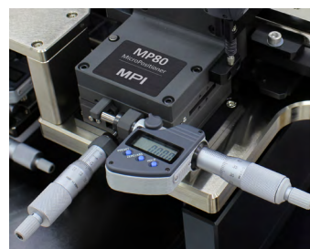
MP80-DXマイクロポジショナ。 X軸のデジタル・マイクロメータ使用
